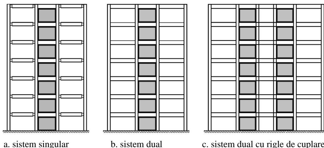
Figura 6.13 Sisteme de cadre cu panouri de forfecare – reprezentare exemplificativă
