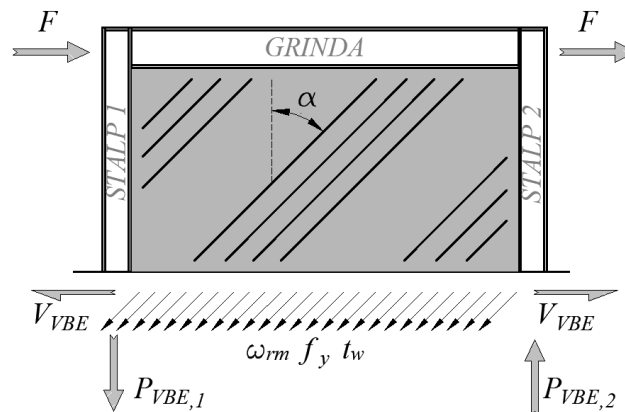
Figura 6.16 Forțele și reacțiunile panoului de forfecare
